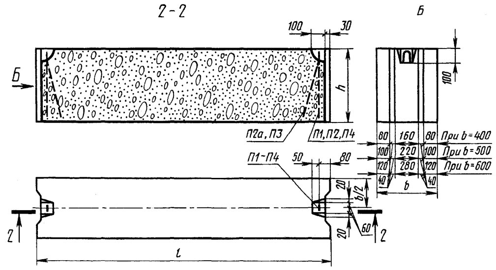
Блоки шириной 400, 500 и 600 мм
